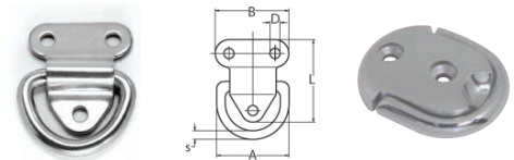
Niroaugbügel mit Basis AISI 304
